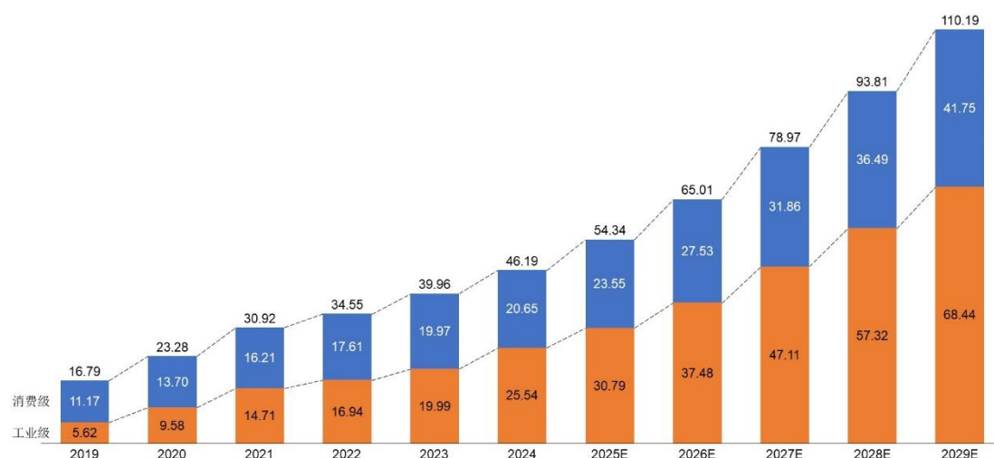
中国工业级及消费级无人机电动力系统市场规模（不含动力电池，亿元）
