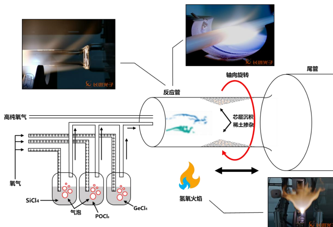
图 5 预制棒制备环节涉及的核心工序
