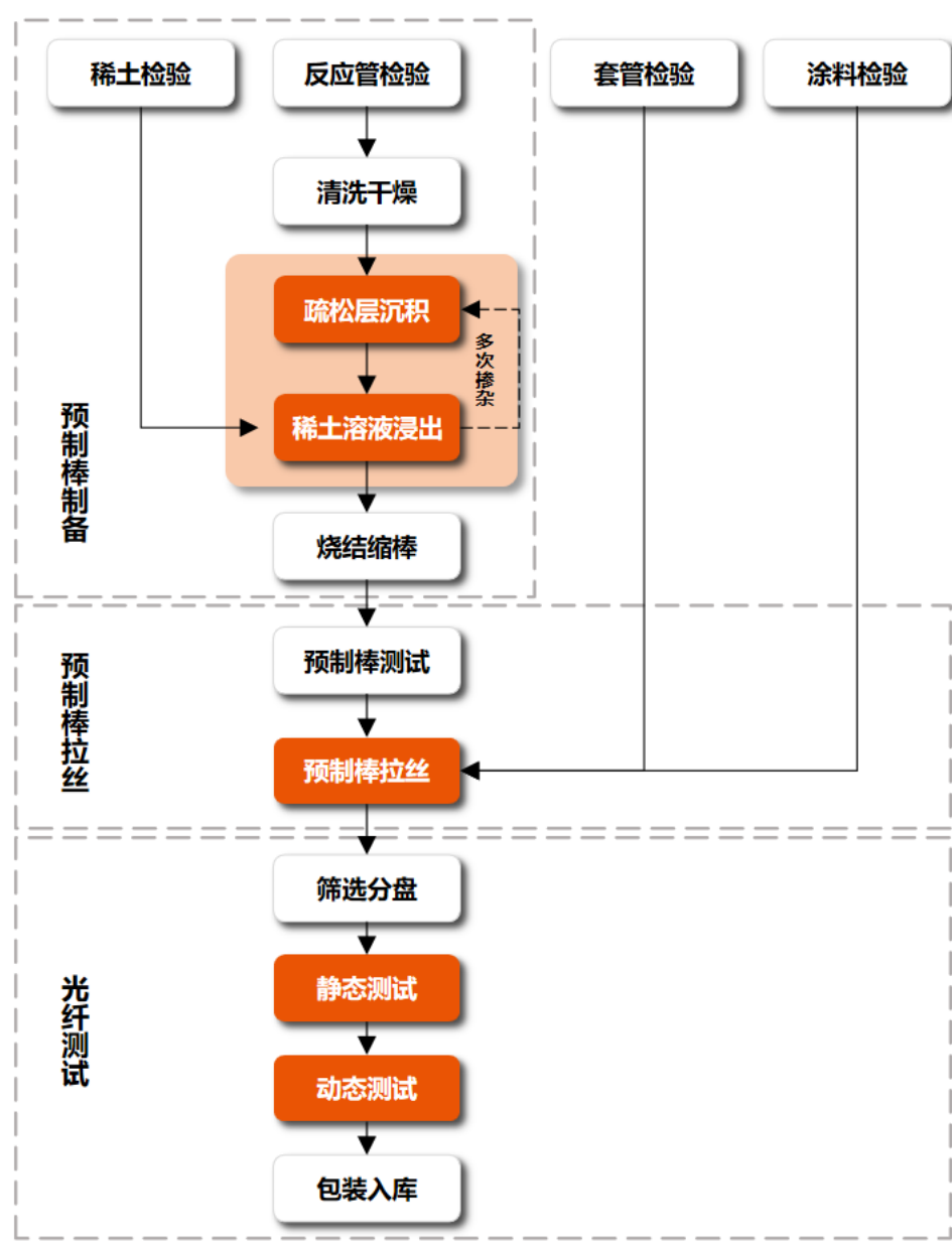
图 4 公司特种光纤生产工艺流程图
