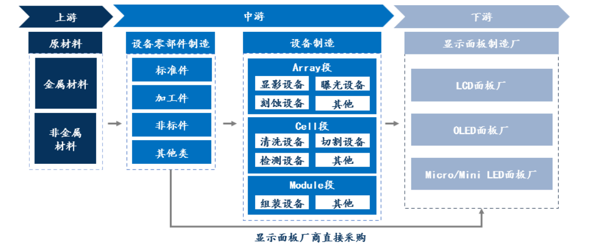
图：显示面板设备零部件行业产业链
