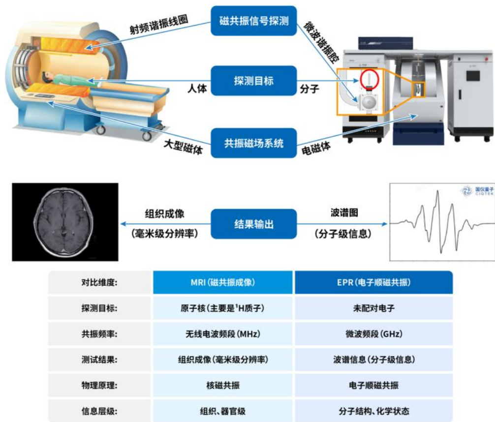
电子顺磁共振波谱仪功能示意图（与核磁共振成像仪器类比）
