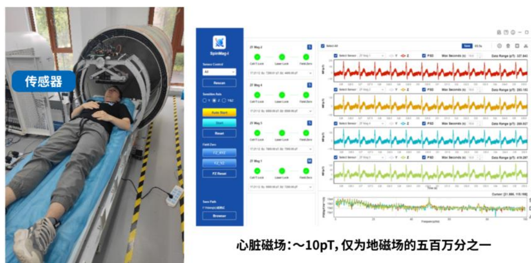
量子自旋磁力仪应用示意图（以检测心脏磁场信号为例）
