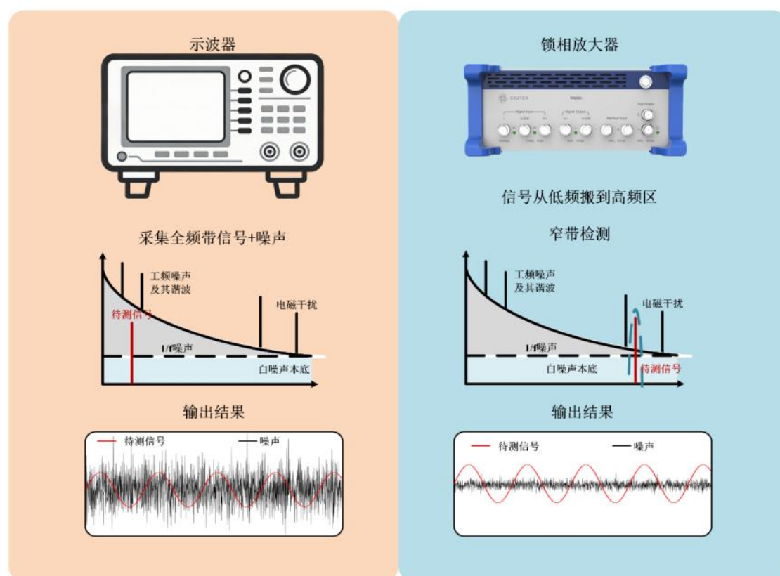
锁相放大器功能示意图（与示波器类比）
