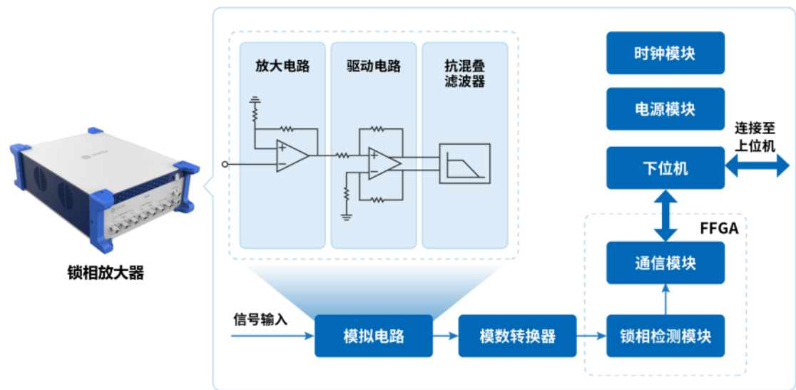
锁相放大器结构示意图
