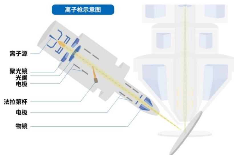
离子枪的结构示意图
