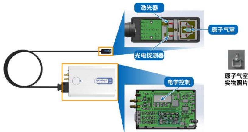
量子自旋磁力仪结构示意图
