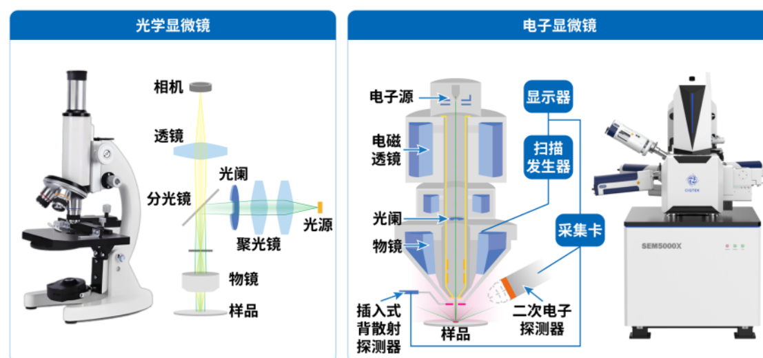
电子显微镜结构示意图（与光学显微镜类比）
