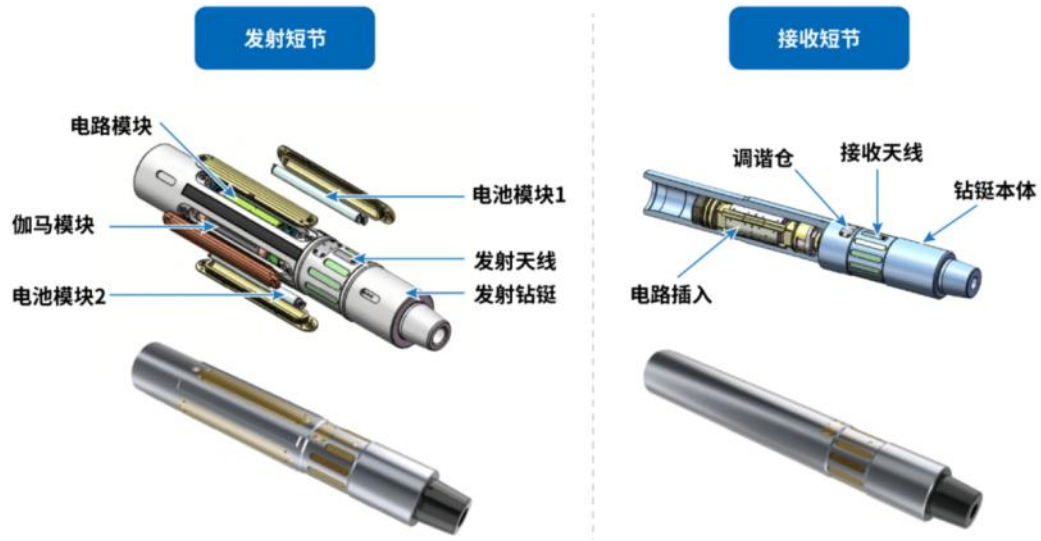
近钻头随钻测量系统结构示意图（包括发射短节、接收短节两部分）
