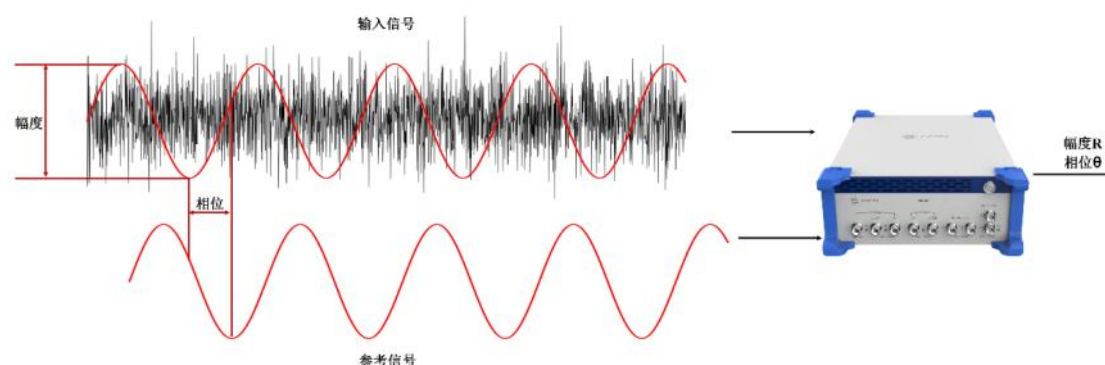
锁相放大器应用示意图（从高噪声的混合输入信号中提取参考信号）
