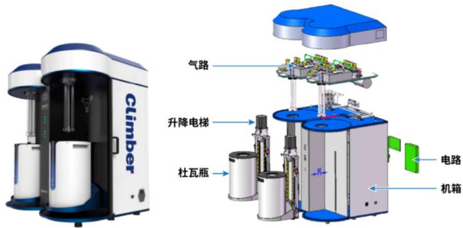
比表面积及孔径分析仪结构示意图
