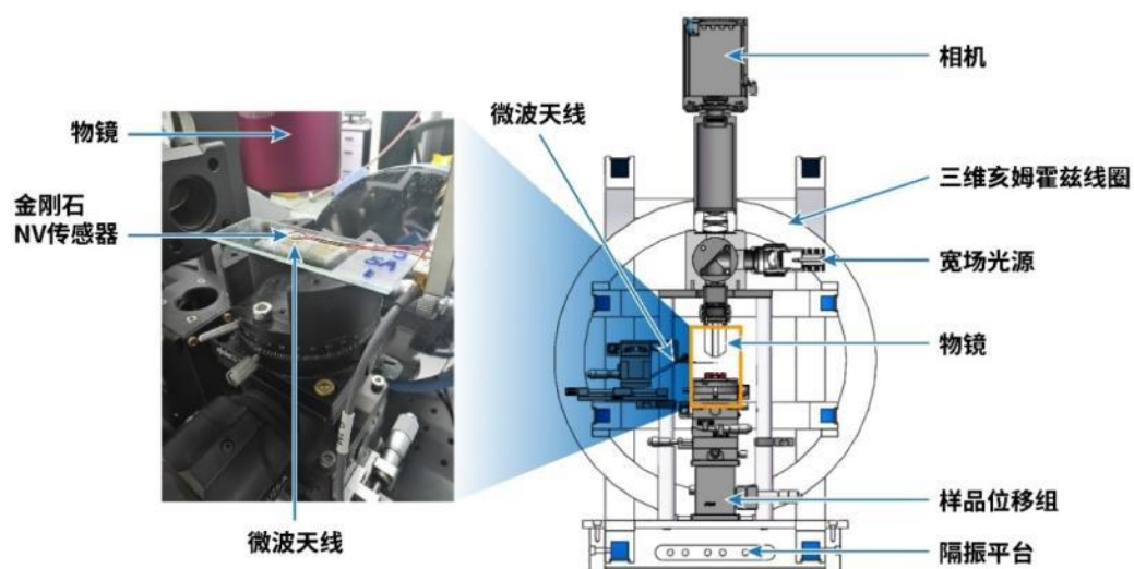
宽场 NV 显微镜结构示意图
