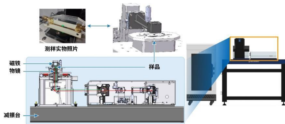
量子钻石单自旋谱仪结构示意图
