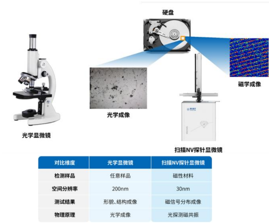
扫描 NV 探针显微镜功能示意图（与光学显微镜类比）
