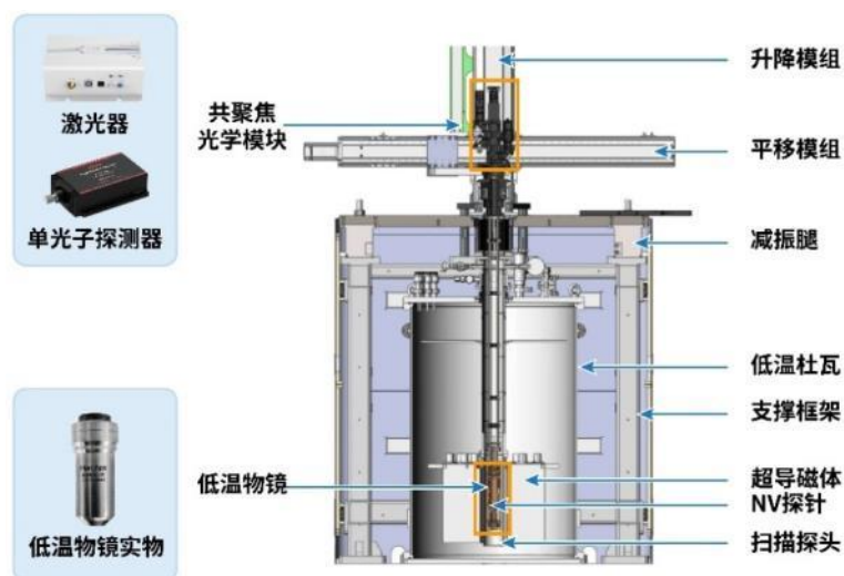
扫描 NV 探针显微镜结构示意图
