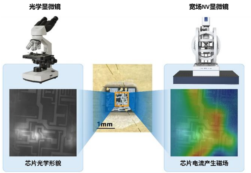
宽场 NV 显微镜功能示意图（与光学显微镜类比）
