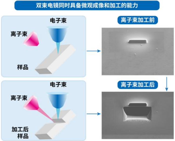
双束电镜的应用示意图（右侧为由电子束观察离子束切削的材料图）
