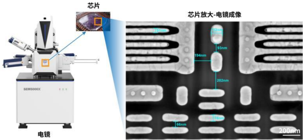
扫描电镜应用示意图（以观察芯片为例）
