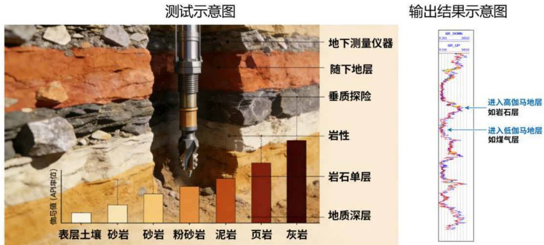
近钻头随钻测量系统应用示意图（输出结果可有效判断地层特性及分布）
